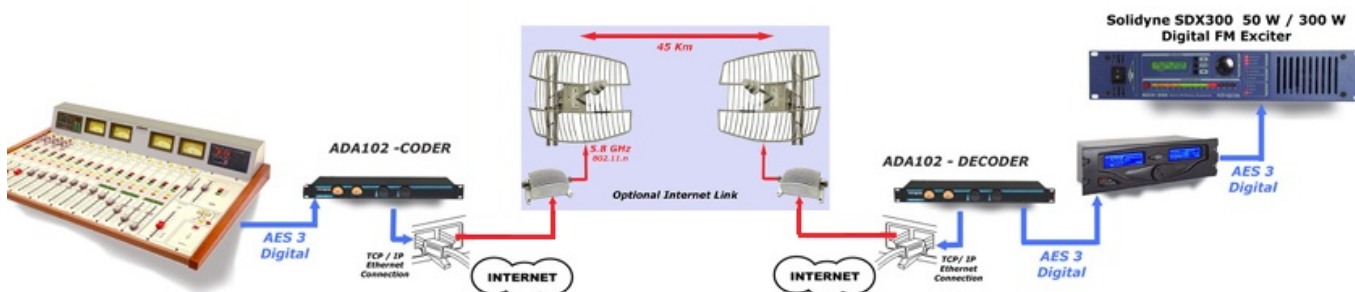
Fig. (b) – Enlace Estudio-Planta usando una cadena de audio digital. Para estaciones de AM, el procesador de audio debe estar próximo al transmisor
