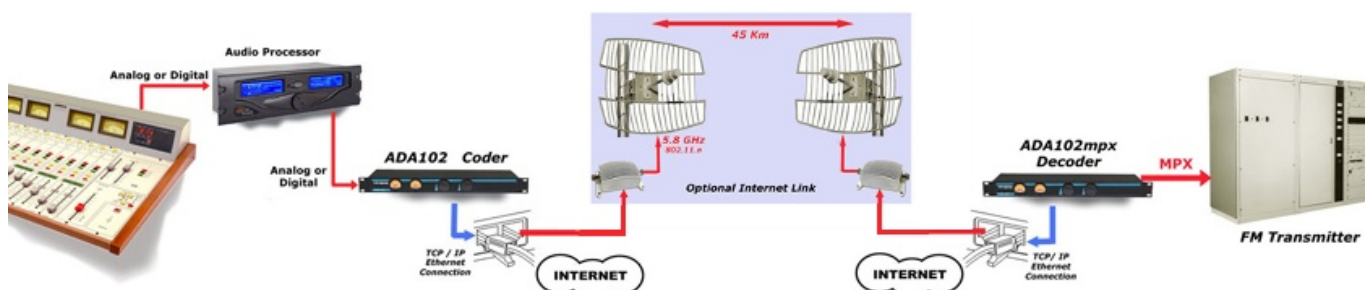
Figura (a) – Enlace Estudio-Planta con el procesador de audio en los estudios
